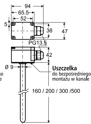
Czujnik prętowy
