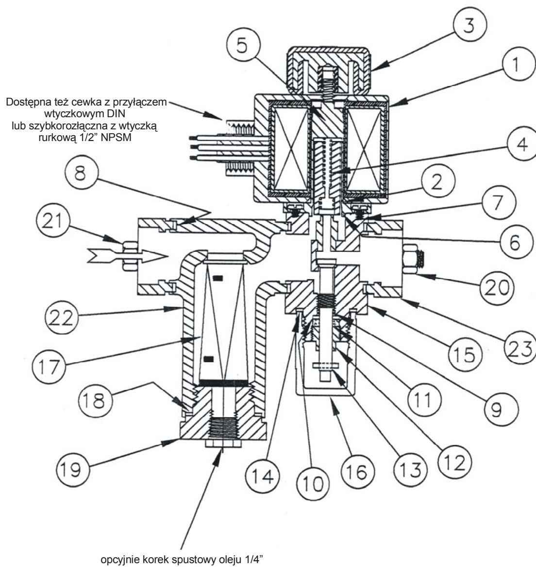
Rysunek zaworu HS6 z filtrem ST050, kołnierzami SW, śrubami.
