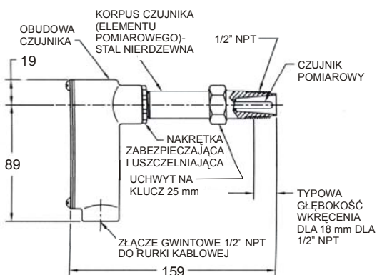
SPS - jednopunktowy czujnik poziomu cieczy
