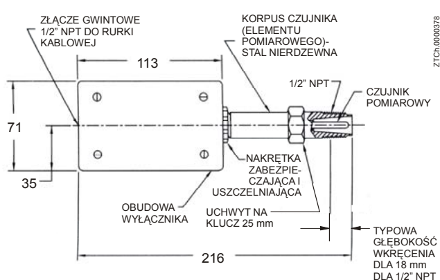
SPS - jednopunktowy wyłącznik poziomu cieczy
