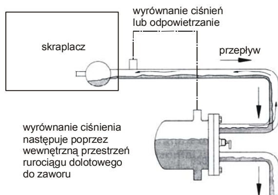
Skraplacz wyparny jednosekcyjny
