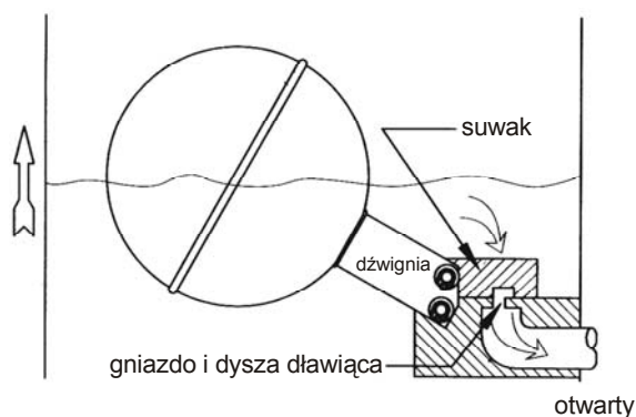
KULA PŁYWAKOWA W POŁOŻENIU GÓRNYM
