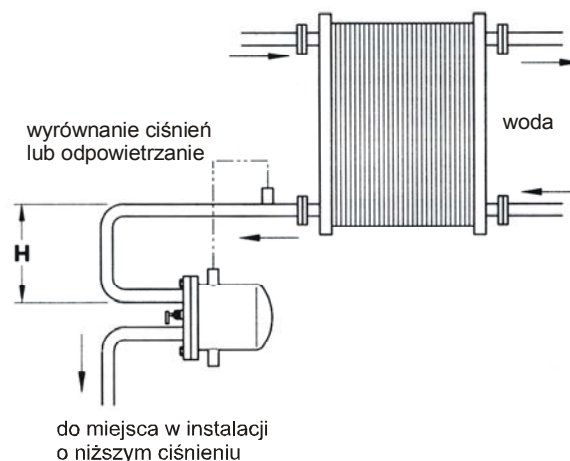
Wymiennik ciepła płytowy (grzanie)
