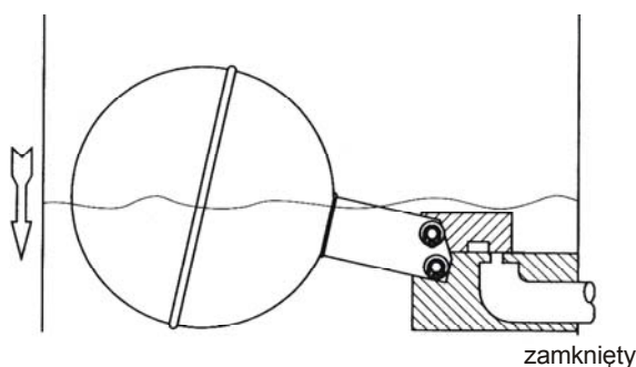
KULA PŁYWAKOWA W POŁOŻENIU DOLNYM
