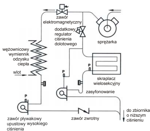
Wymiennik wężownicowy odzysku ciepła
