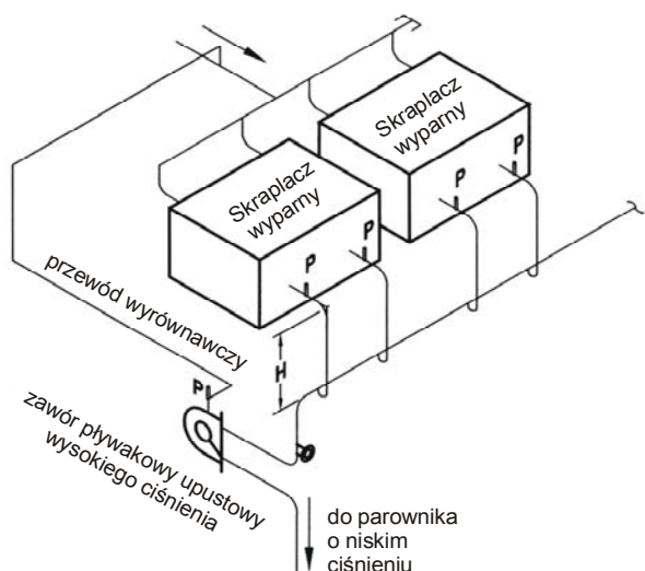
Skrapłacz wielosekcyjny
