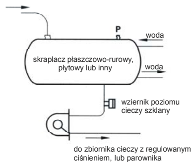
Skraplacz chłodzony wodą
