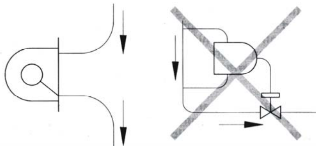
Zawór pływakowy upustowy cieczy Hansena
